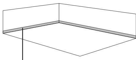
ARDEX DS 70 MC Isolation Périmétrique Bande
