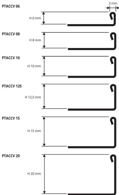
ACIER INOX AISI 304/1.4301-V2A POLI avec film de protection longueur b. 2,7 ML - cond. 20 Pces - 54 ML - 10/10 mm
