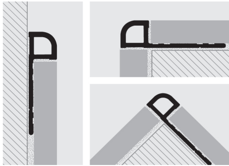
ALU. BRONZE ANCIEN ANODISÉ BROSSÉ thermo packed - longueur b. 2,7 ML - cond. 40 Pcs - 108 ML
