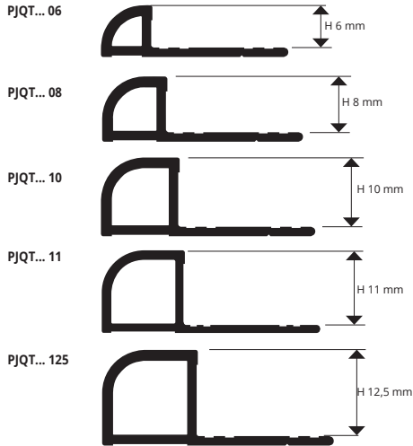
ALUMINIUM BROSSÉ (ARGENT) thermo packed - longueur b. 2,7 ML - cond. 40 Pcs - 108 ML (H 12,5 mm, 15 mm - cond. 20 Pcs)
