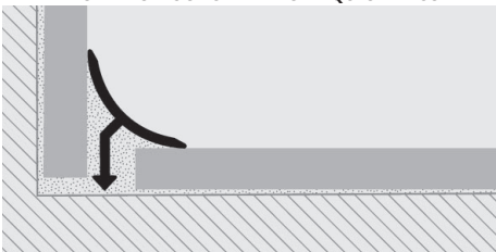
LAITON POLI ET CHROMÉ thermo packed longueur b. 2,7 ML - cond. 40 Pcs - 108 ML
