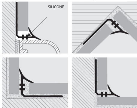
RACCORDS ANGLES INTERNES-EXTERNES-TROIS VOIES ALUMINIUM ANODISÉ ARGENT et OR - cond. 2 Pcs
